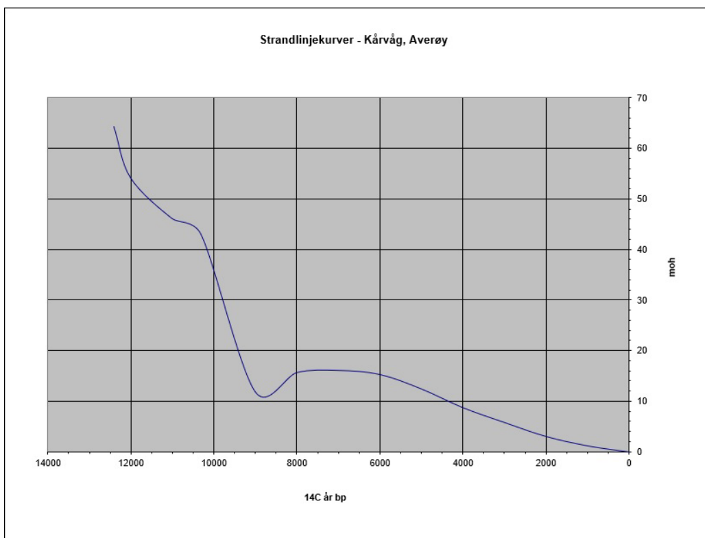
Figur 5. Strandlinjekurve for Kårvåg, i Averøy kommune etter skjema utarbeidet av David N. Simpson, mars 2001 (jfr. Svendsen & Mangerud 1987, Bondevik, Svendsen og Mangerud 1998).
