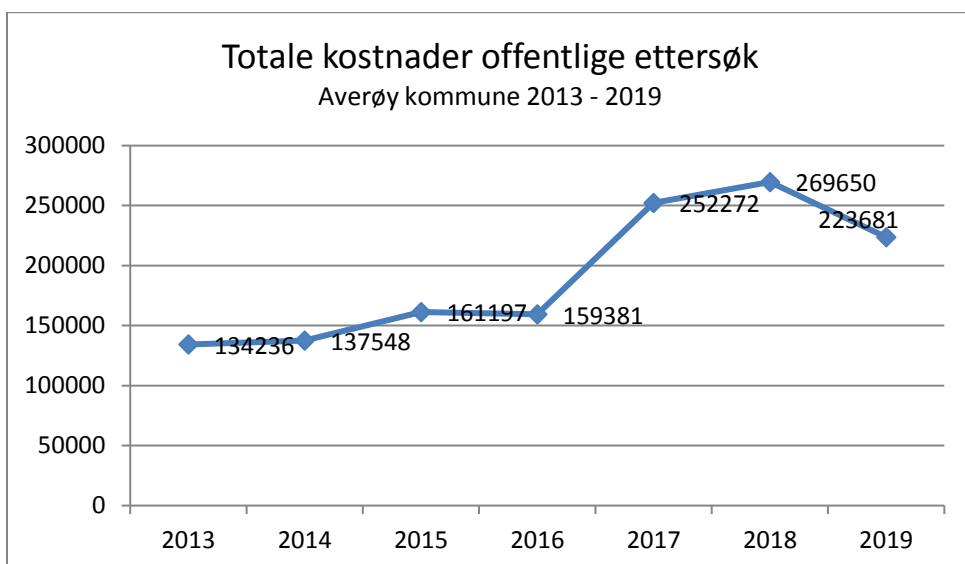
Figur 8. Totale kostnader for offentlige ettersøk. Averøy kommune i perioden 2013-2019.
