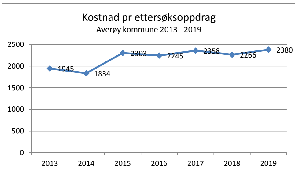
Figur 9. Kostnad pr ettersøksoppdrag. Averøy kommune i perioden 2013-2019.
