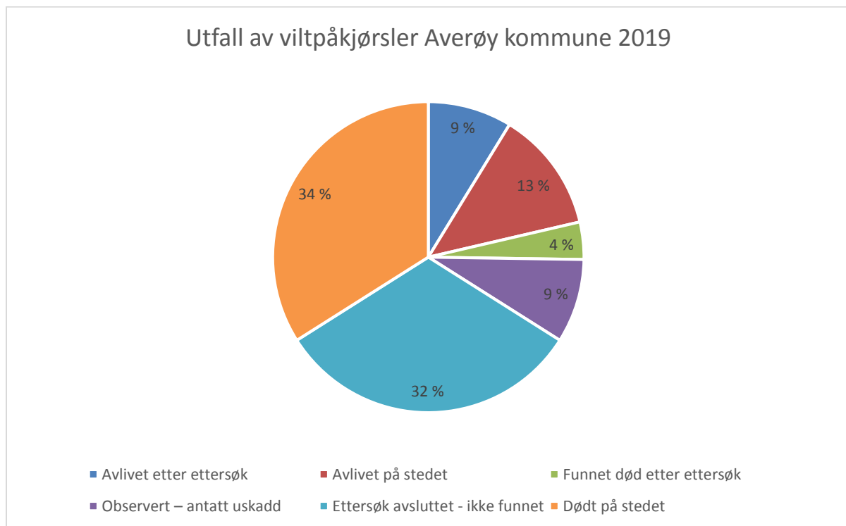
Figur 6. Utfall av viltpåkjørsler i prosent. Averøy kommune i perioden 01.01.2019-31.12.2019.
