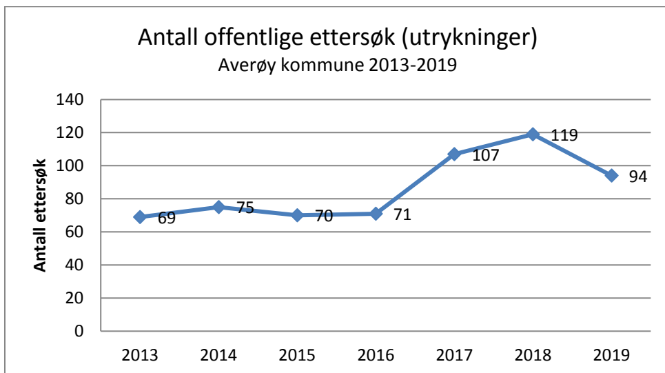
Figur 7. Antall utførte kommunale ettersøk. Averøy kommune i perioden 2013 - 2019.
