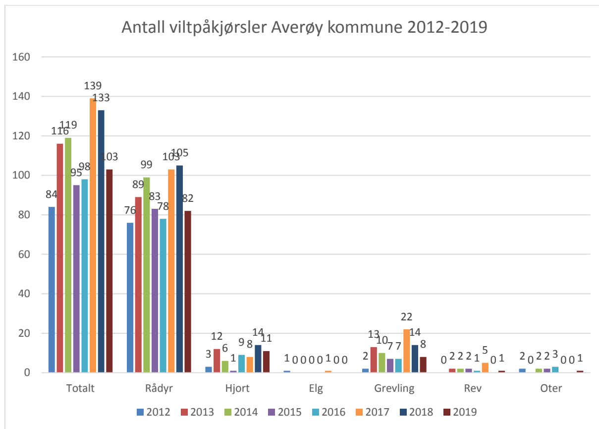
Figur 1. Utvikling i antall registrerte viltpåkjørsler i Averøy siste 7 år. F.o.m. 1.januar til og med 31. desember.
